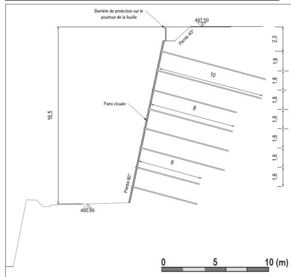
Coupe type du confortement réalisé, longueur 130 m.
